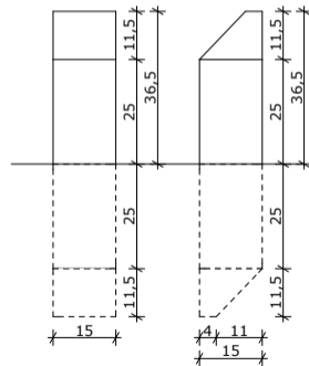
marco hectométrico
