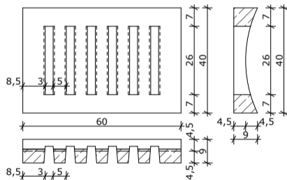
grelha sumidouro / sarjeta
